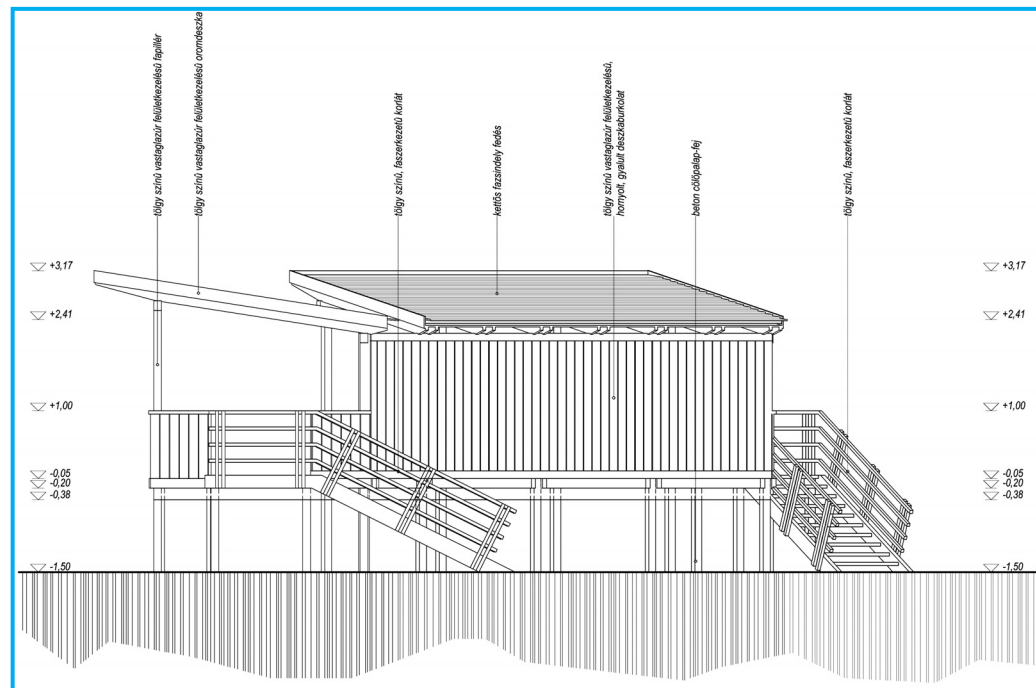
Madárles - E-07 északi homlokzat
